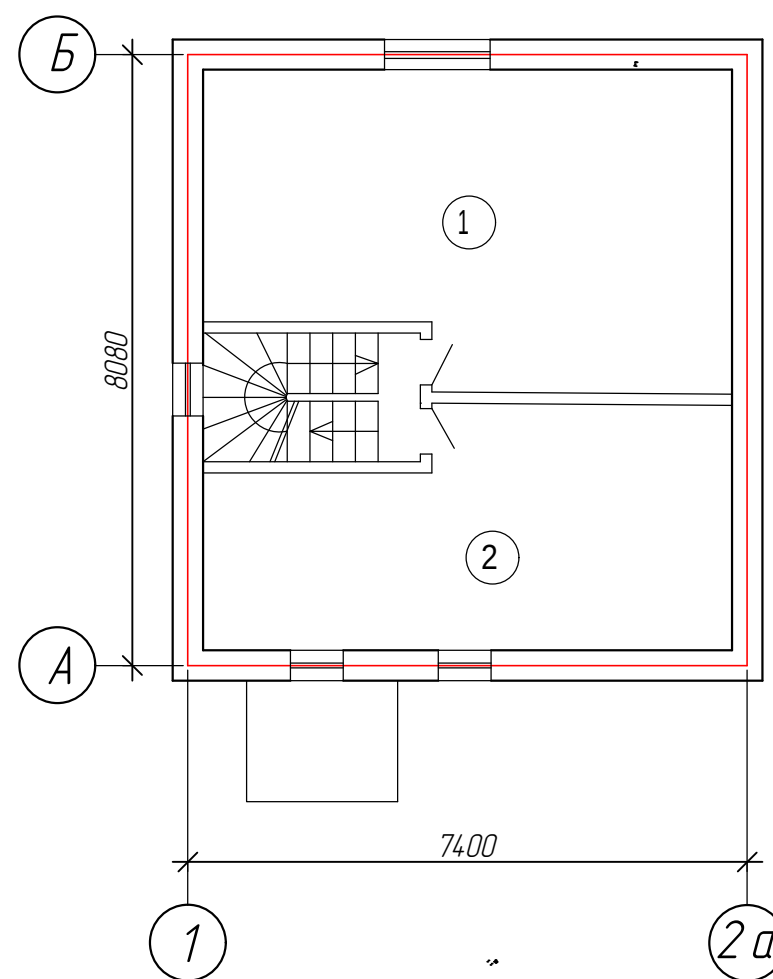
План мансардного этажа
